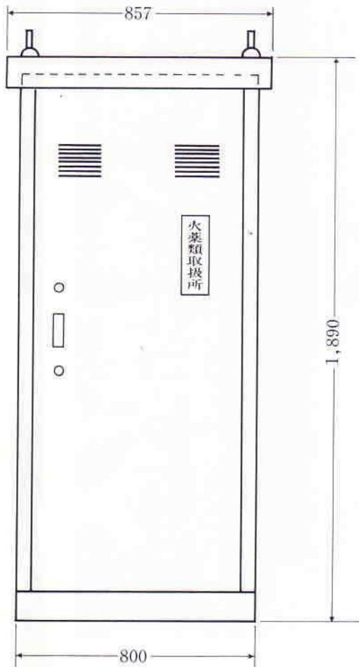
正面図
