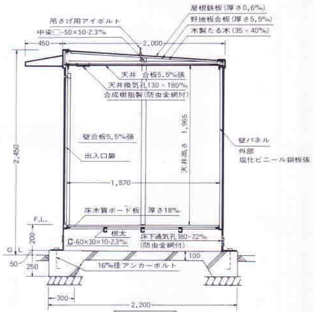
矩計詳細図
