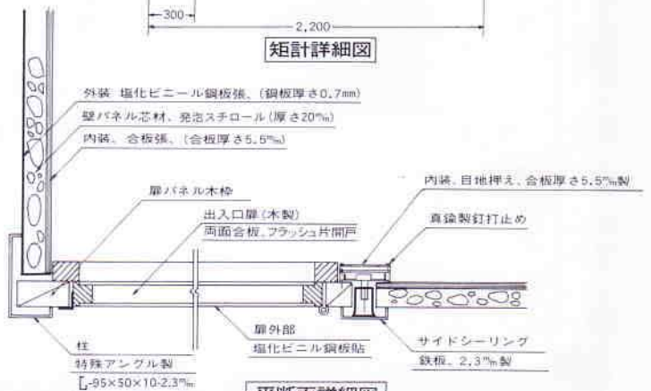
平断面詳細図
